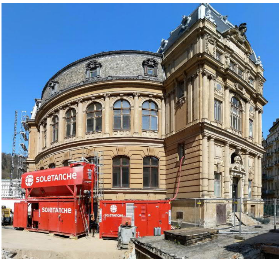
Zařízení staveniště a rekonstruovaný objekt
