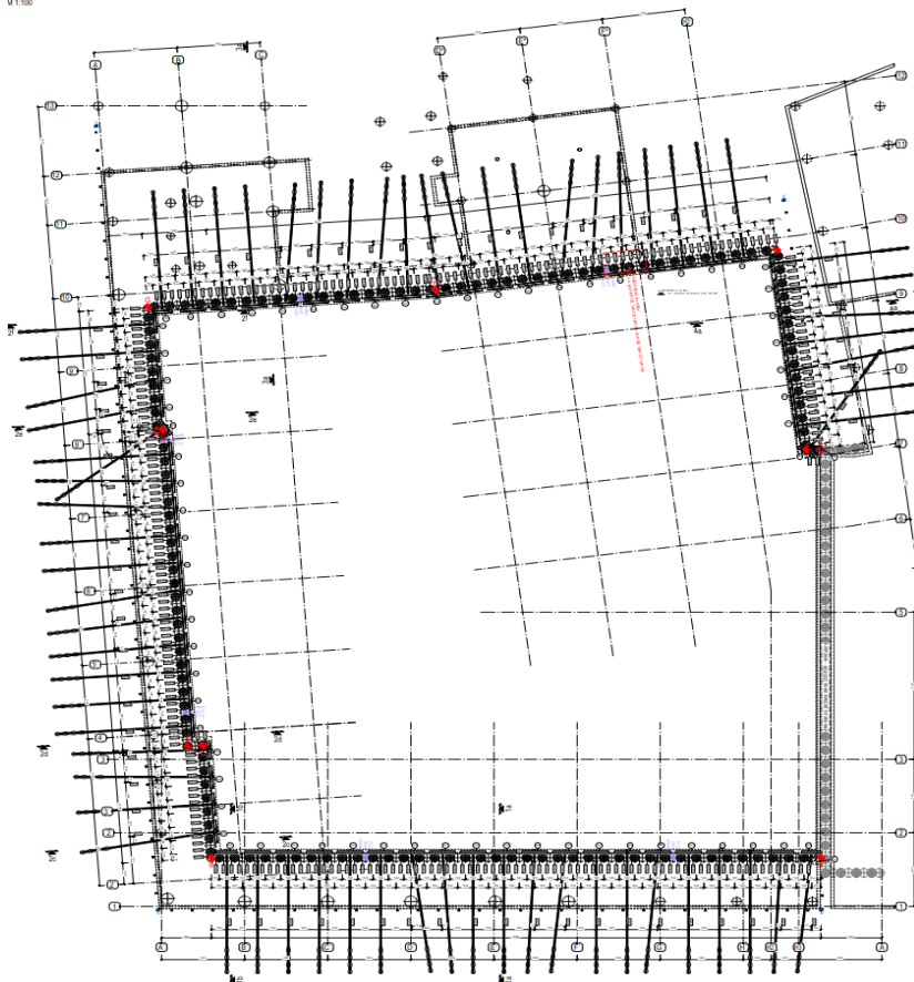
DOCK 5 - půdorys tesniacej a pažiacej steny
