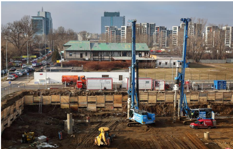
Zajištění jámy kotvenou záporovou stěnou
