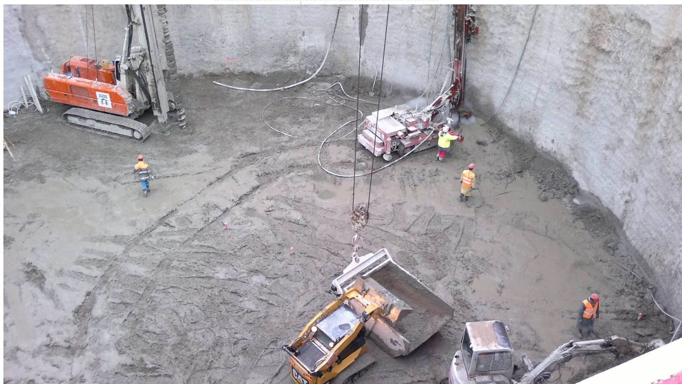
Pohled do stavební jámy – provádění tryskové injektáže a předvrtů
