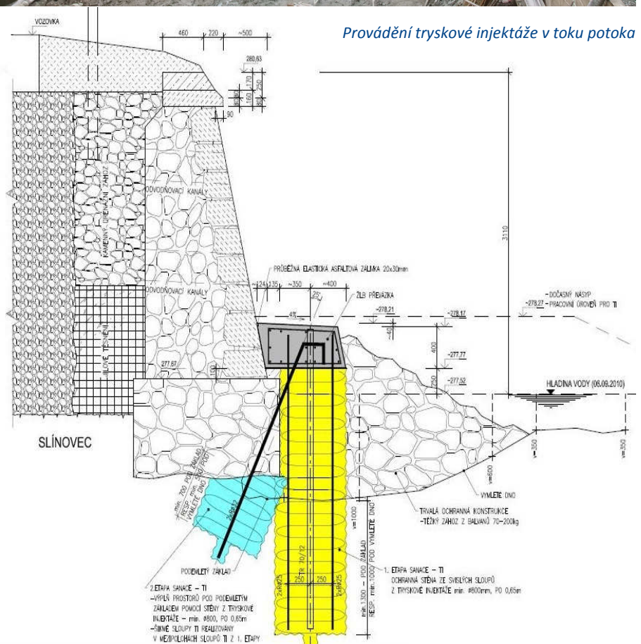
Půdorys a řez – sanace stávající kamenné opěrné zdi
